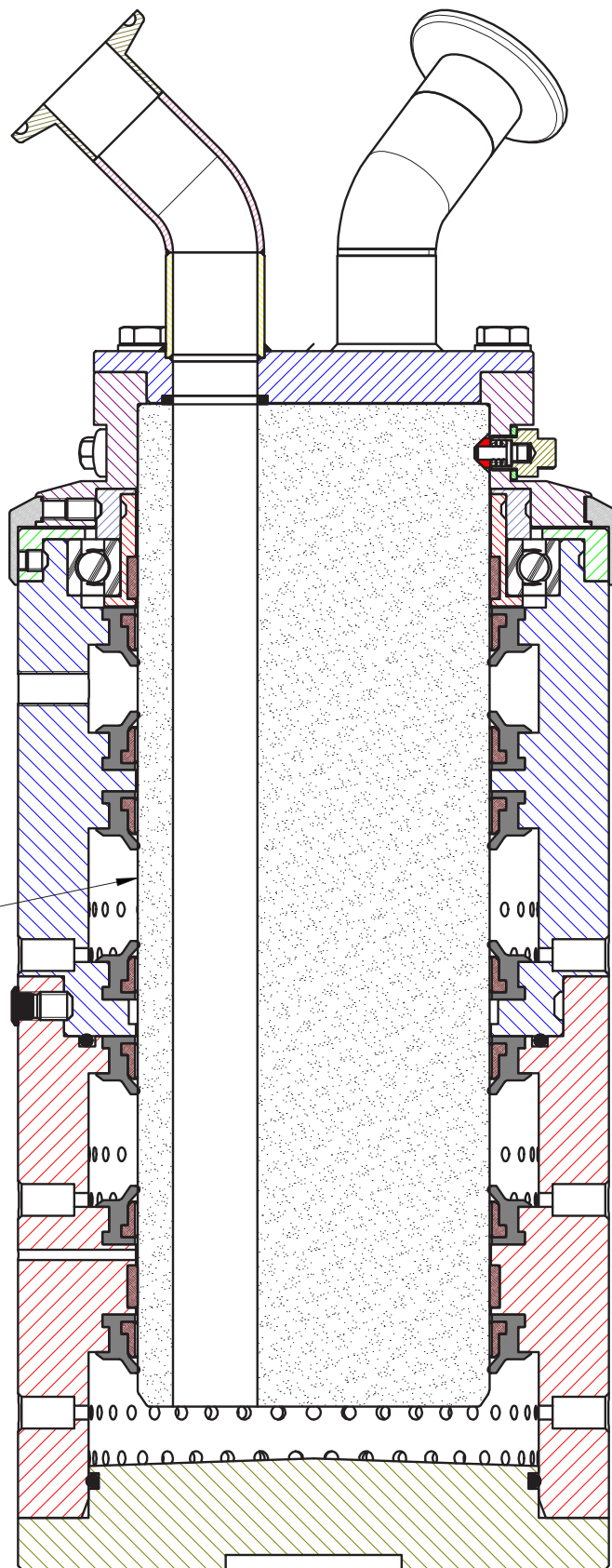
SEZIONE COLLETTORE 80/80/80 USCITE + passaggio aria
