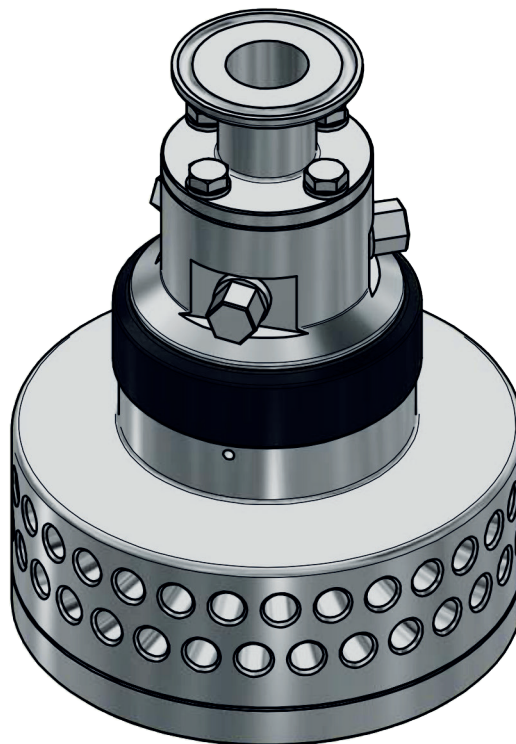
COLLETTORE PER RISCIAQUATRICE DA 40 A 100 USCITE
