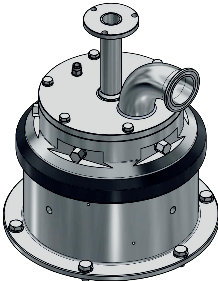
COLLETTORE PER RIEMPITRICE FINO A 30 USCITE DA 3/4" (ENTRATA DN40) COMPLETO DI PASSAGGIO INTERNO PER CAVI ELETTRICI
