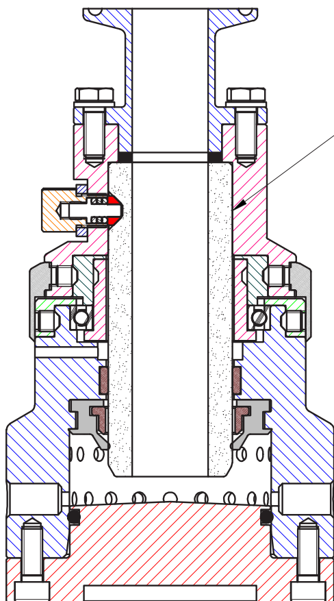
SEZIONE COLLETTORE 20/40 USCITE
