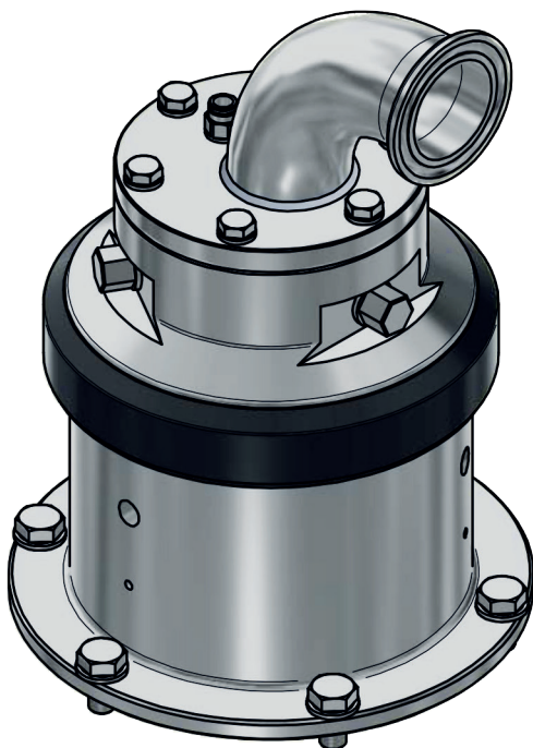
COLLETTORE PER RIEMPITRICE FINO A 30 USCITE DA 3/4" (ENTRATA DN40)
